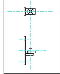
組立図 146.04.015+141.04.015
