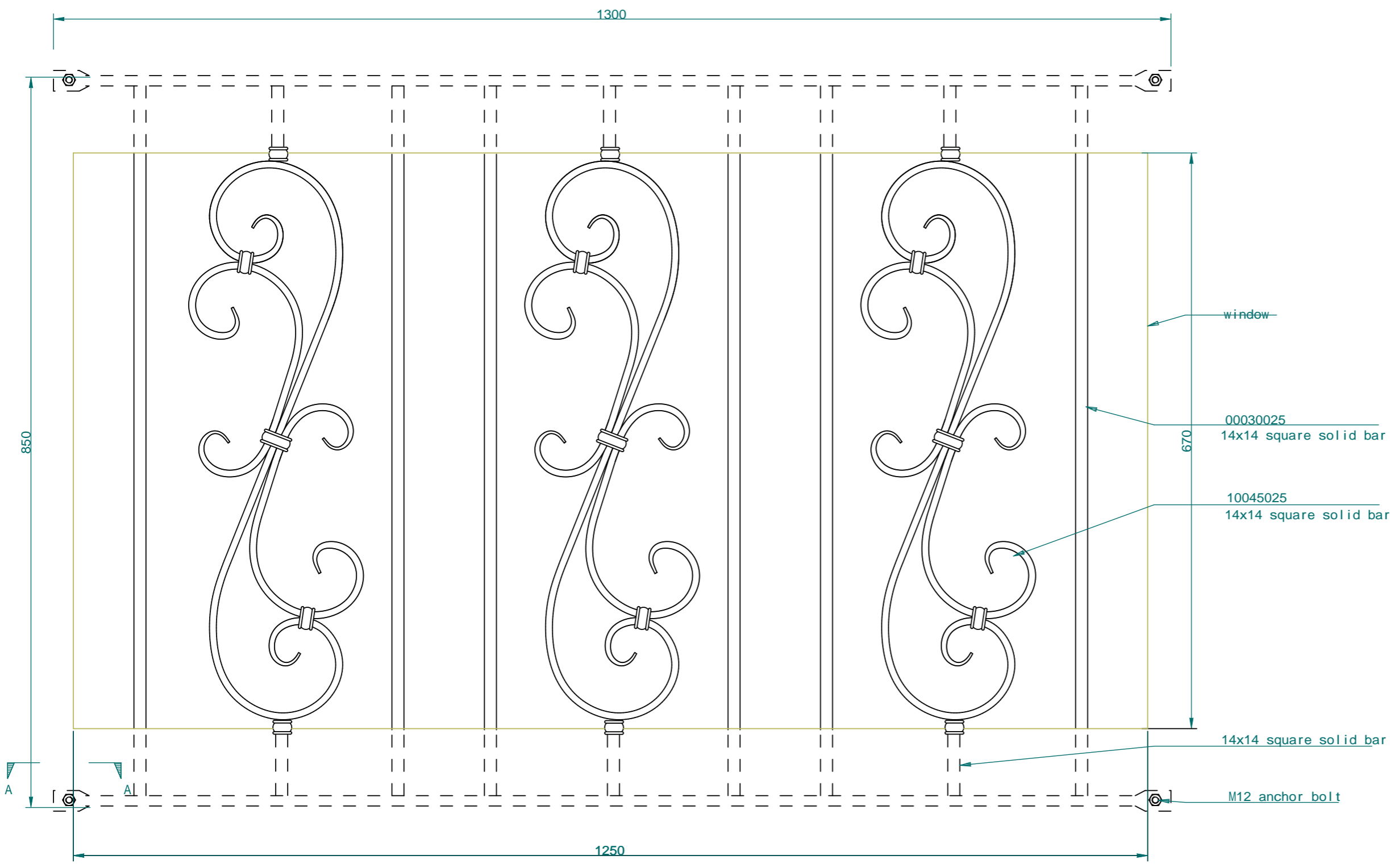
ELEVATION 1:5
