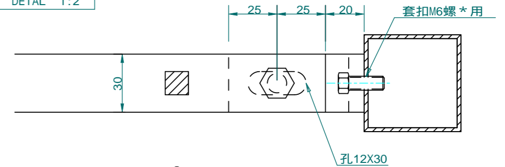
DETAL 1:2
