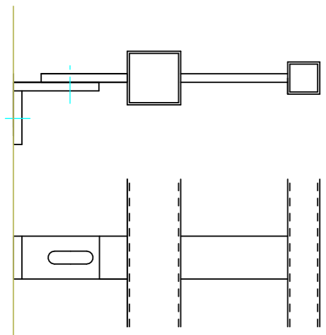
壁付部詳細 1:5
