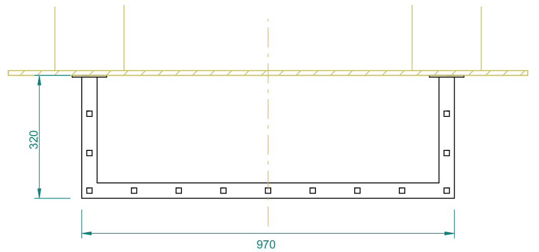
B-B
