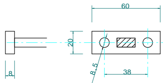
DETAIL A 1:2 DETAIL B 1:2
