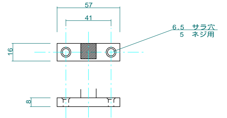
取付ベース詳細 1:2
