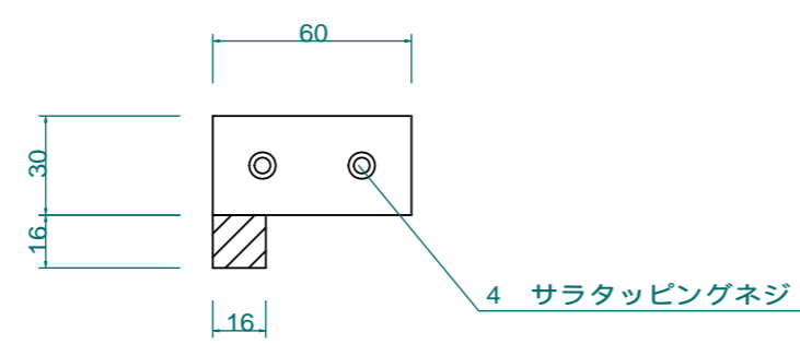
取付部C詳細 S=1:4
