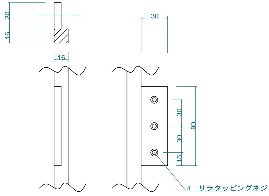
取付部A詳細 S=1:4
