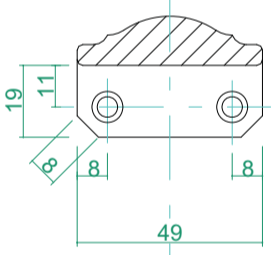
壁付け金具詳細 1:2
