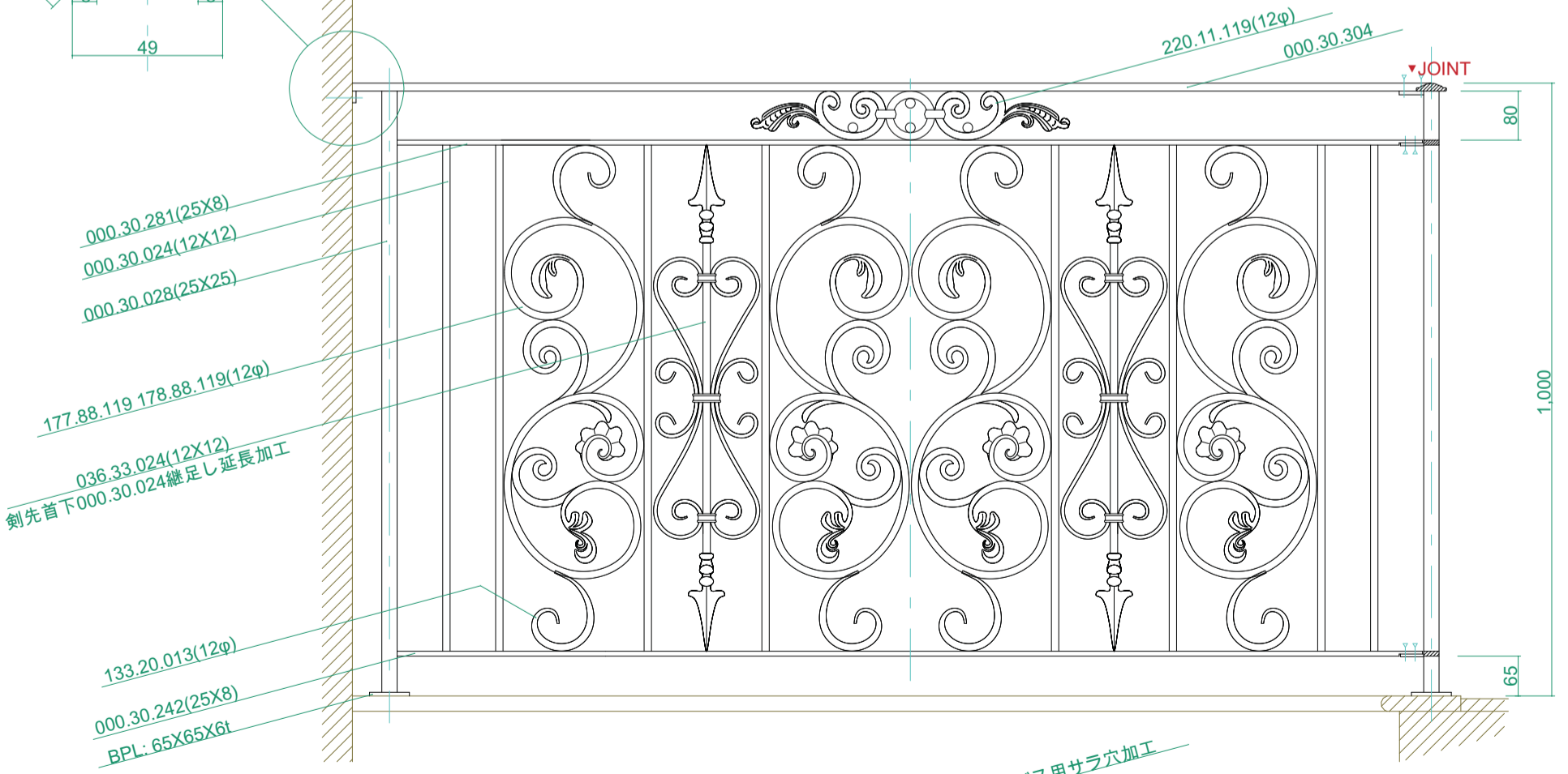
ジョイント部詳細1:2
