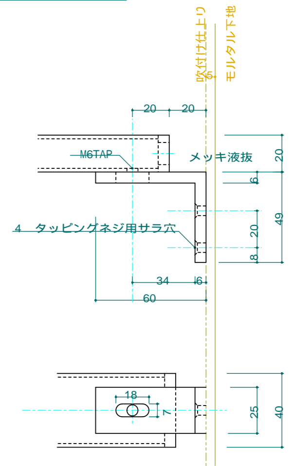
取付金具詳細 1:2
