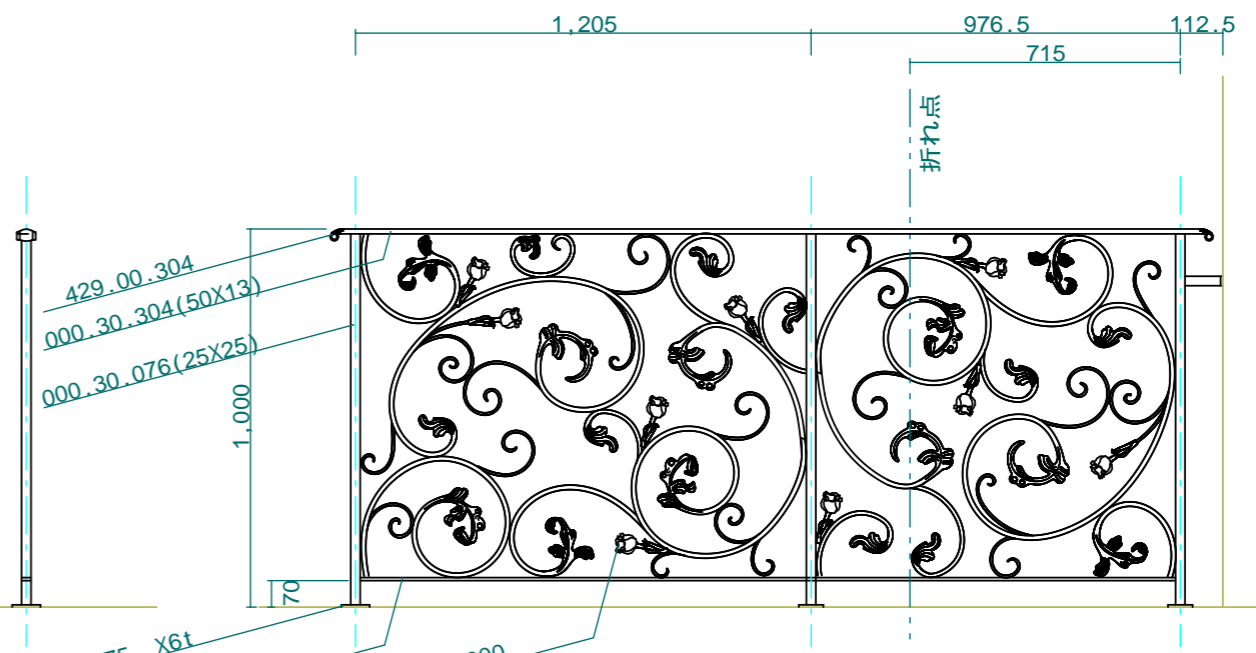
B-B (R部展開寸表示)
