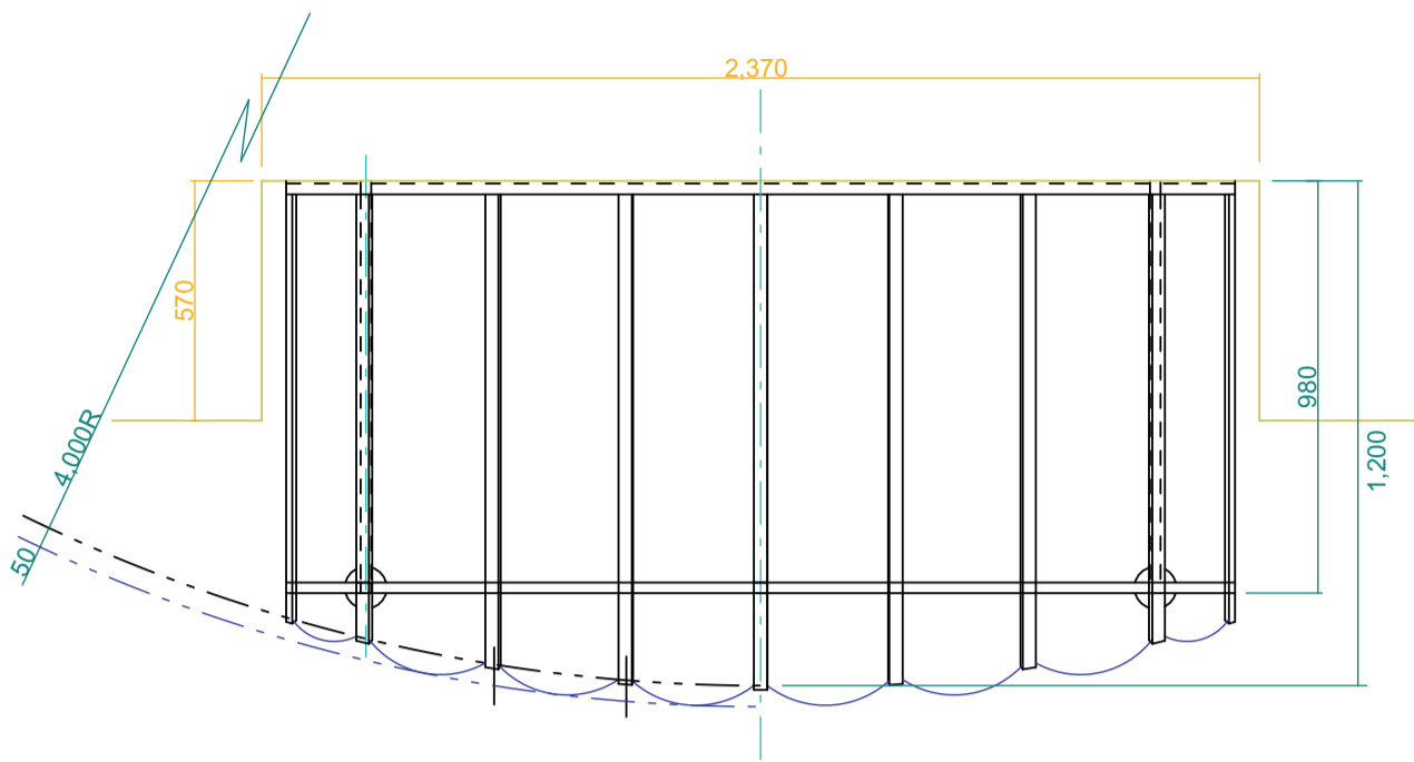
屋根板止め桟詳細 1:3
