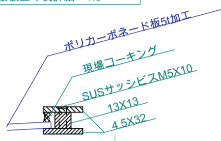
屋根板止め桟詳細 1:3
