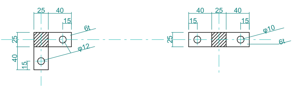
床付ベースプレート詳細 1:4
