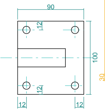
ピボットヒンジ受け詳細 1:3
