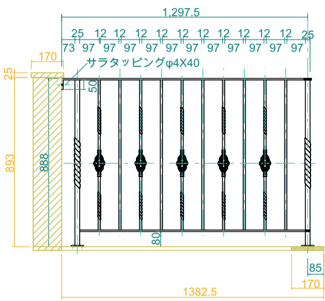
A-A
