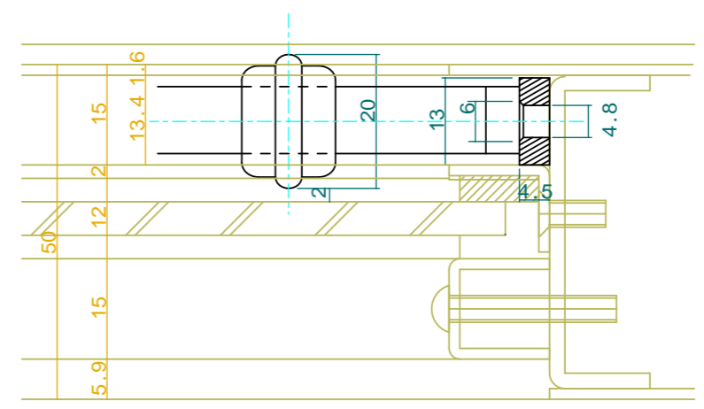
取付サラ穴詳細 1:1 (パーツ納まり検証図)
