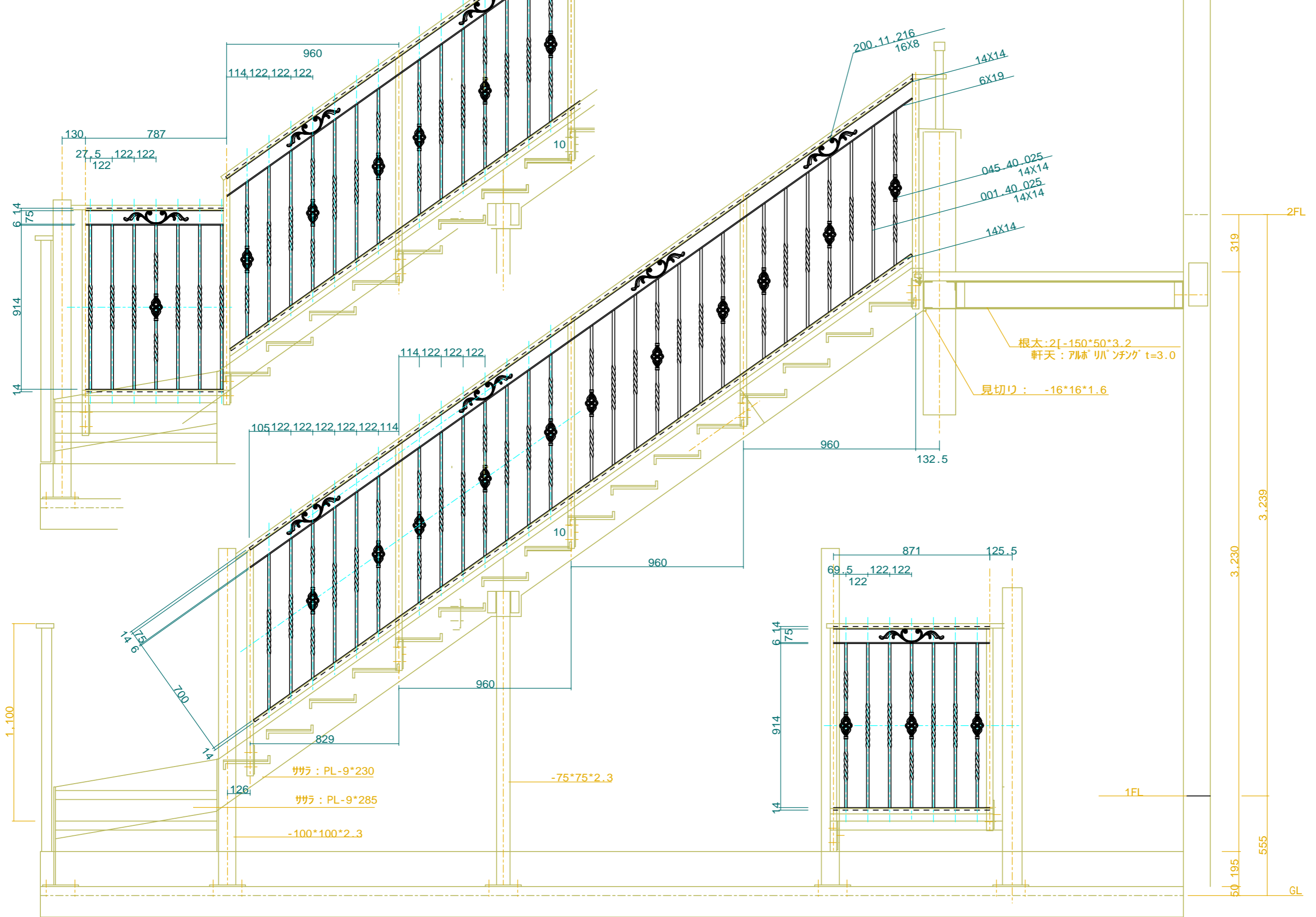
廻り段: PL-4.5箱曲げの上 成形板
