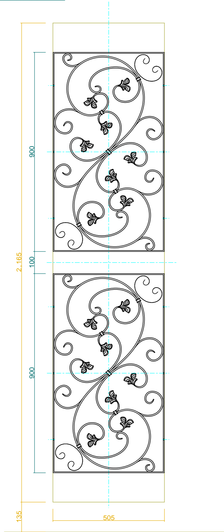
取付姿図 1:10
