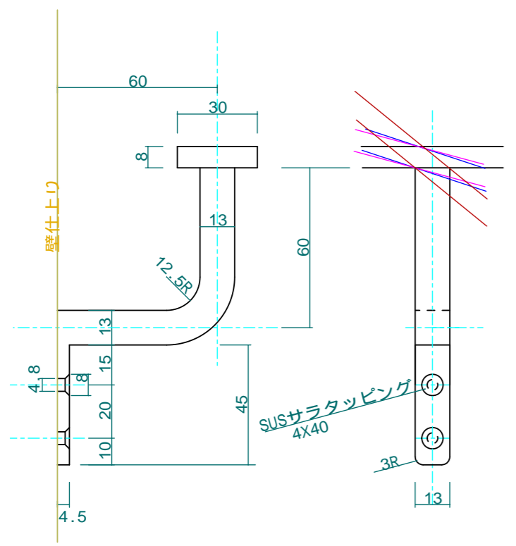
ブラケット詳細 Scale=1:2
